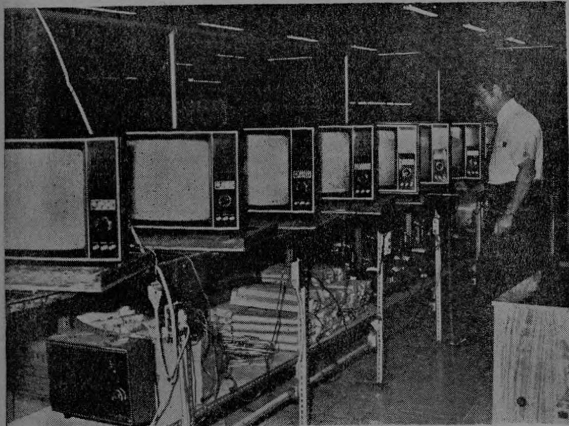
El Ing. Belamarich, haciendo la prueba final de calidad de los televisores GENERAL ELECTRIC, fabricados bajo licencia, por INELCO.
